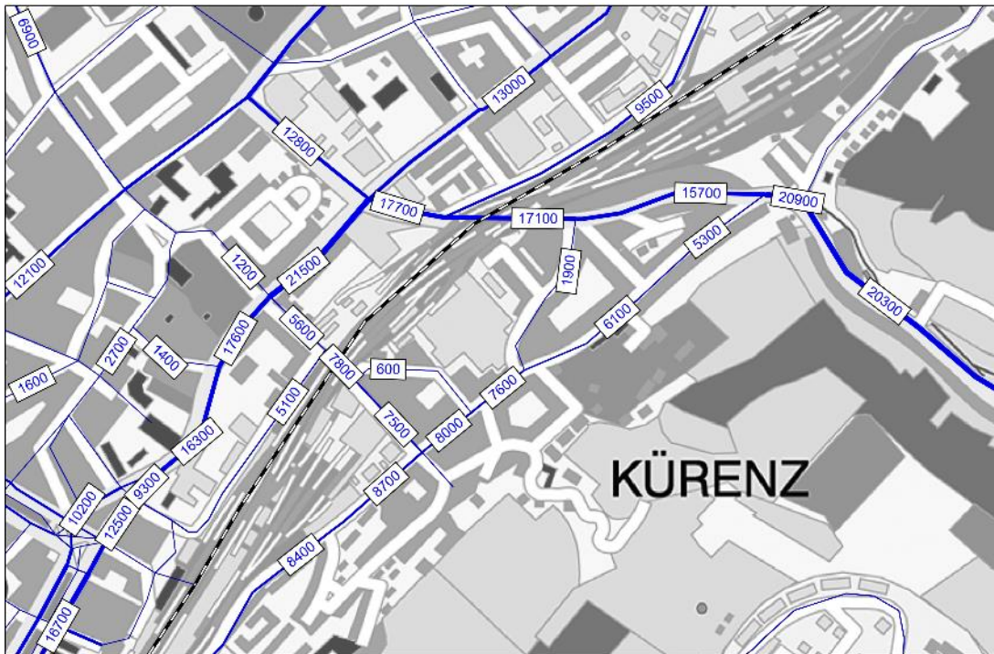
Abbildung 10: Kfz-Verkehrsmengen im Ist-Zustand (DTVw)
